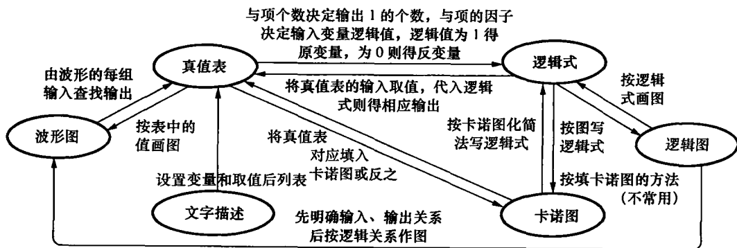
图 1.1.5 六种逻辑表示方式的转换路径
