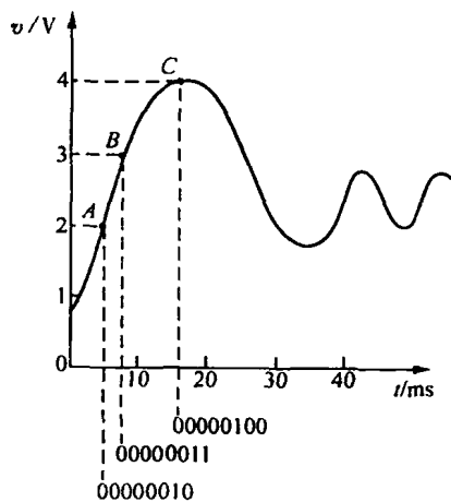
图 1.1.4 模拟电压信号变换成数字代码
