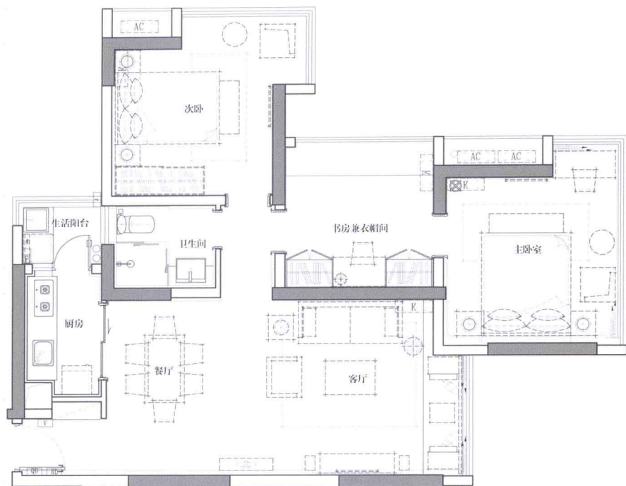
平面布局图
