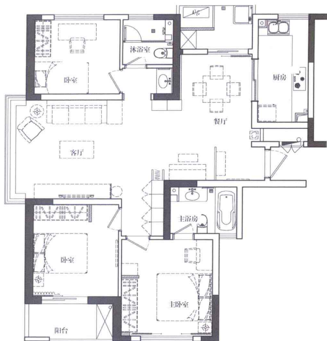
平面布局图
