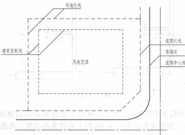
图 1-1-1 基地各种控制线
