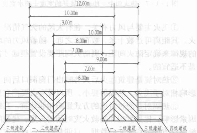
图 1-1-5 民用建筑之间的防火间距
