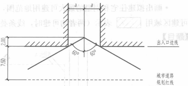
图 1-2-1 汽车库库址车辆出入口通视要求 a—视点距出入口两侧距离
