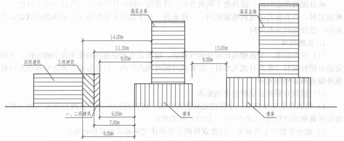
图 1-1-6 高层建筑之间及高层建筑与其他民用建筑之间的防火间距
