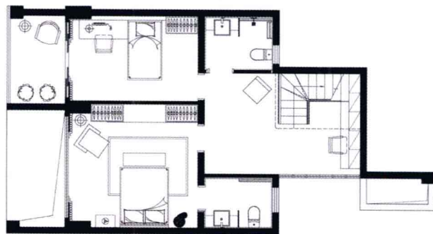
二层平面布置图
