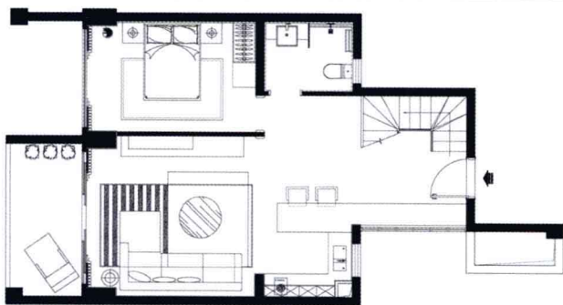
一层平面布置图
