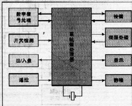
图2-10 汽车CD激光唱机的控制系统框图
