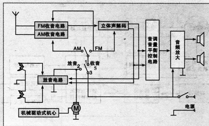
图2-5 汽车收、放音机框图
