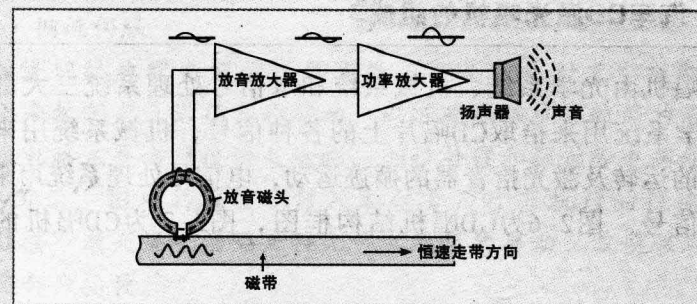
图2-4 磁带放音原理
