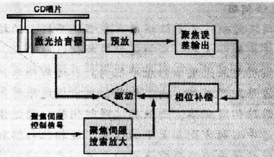
图2-8 CD唱机的聚焦伺服电路
