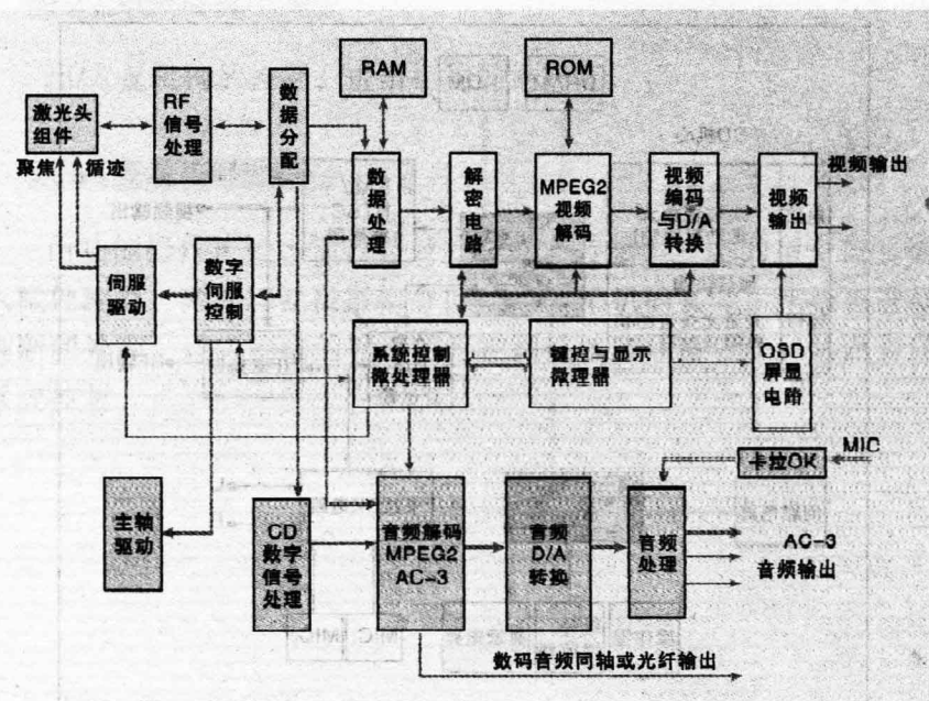
图2-12 DVD的结构
