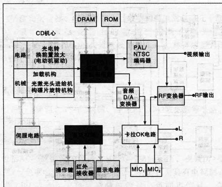
图2-11 VCD影碟机的基本构成
