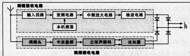
图2-1 汽车收音机（调谐器）的电路框图
