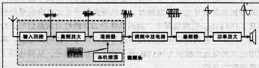
图2-3 调频收音机的电路框图及信号波形的变化
