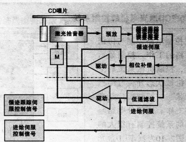
图2-9 CD唱机的循迹和进给伺服电路
