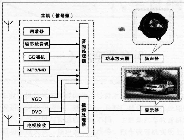
图1-2 汽车多媒体的基本组成
