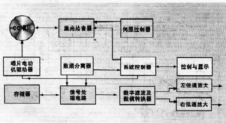
图2-6 CD唱机结构框图
