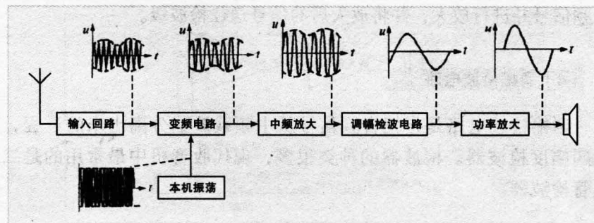
图2-2 调幅收音机的电路框图
