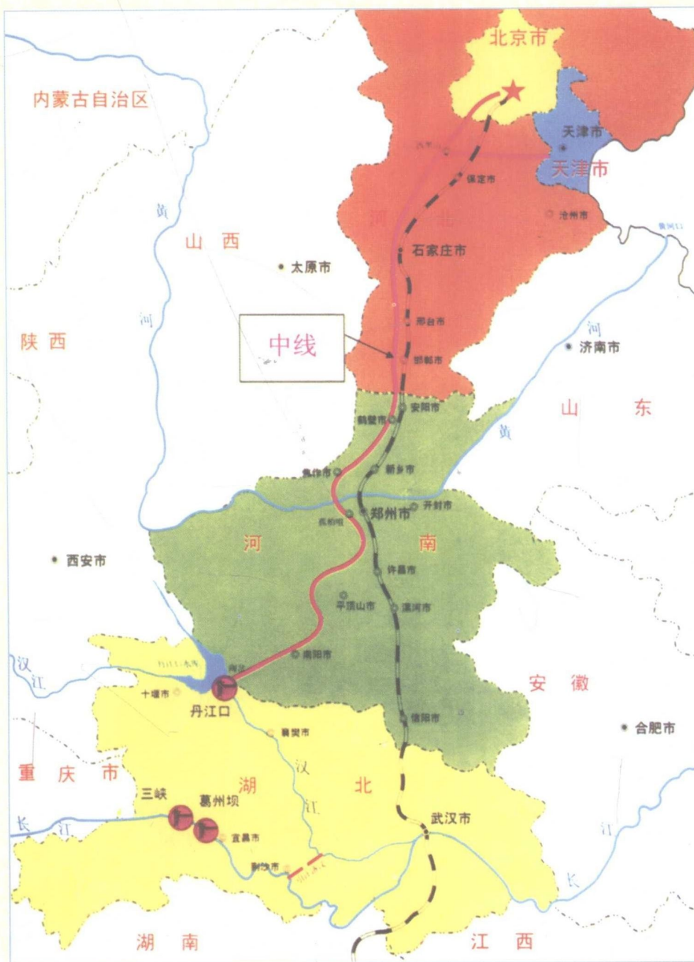
南水北调中线工程示意图
