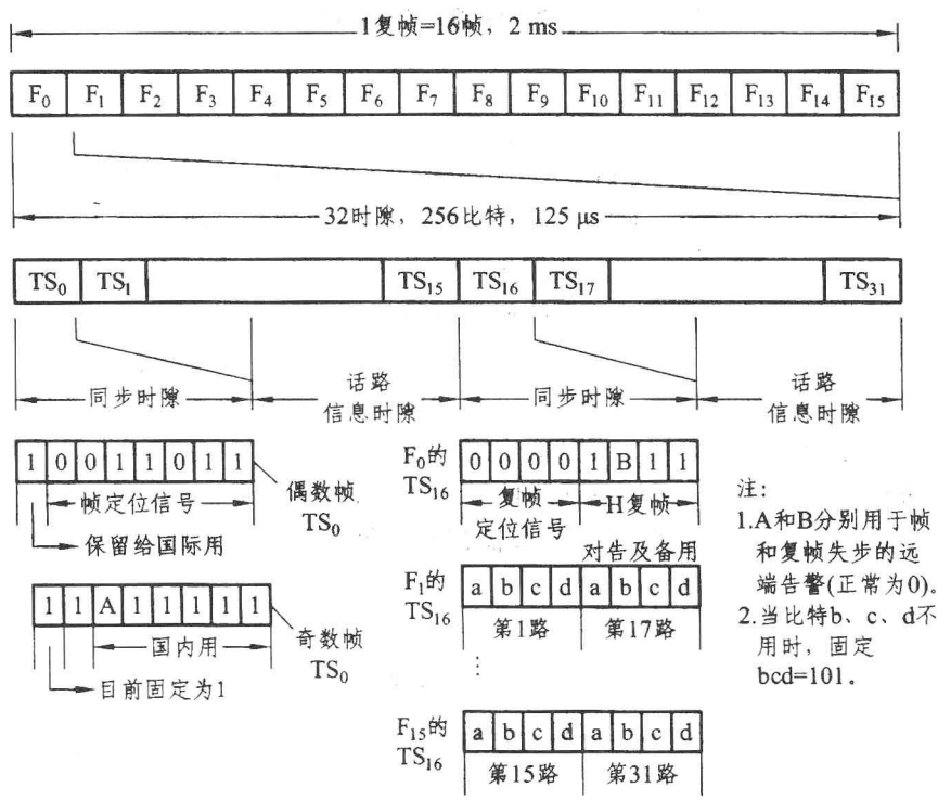
图 1.8 30/32 路 PCM 系统的帧结构
