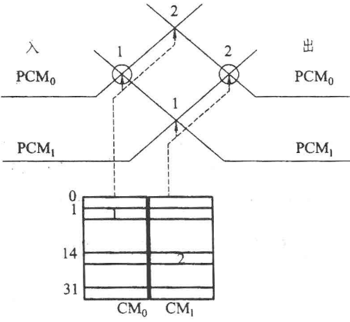
图 1.10 S 接线器结构示意图
