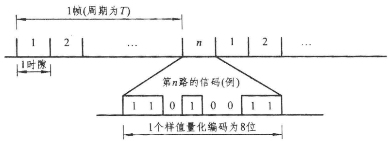
图 1.5 时分多路复用示意图
