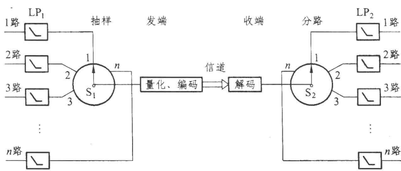
图 1.6 时分多路复用电路结构图
