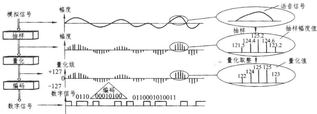
图 1.2 脉冲编码调制过程示意图
