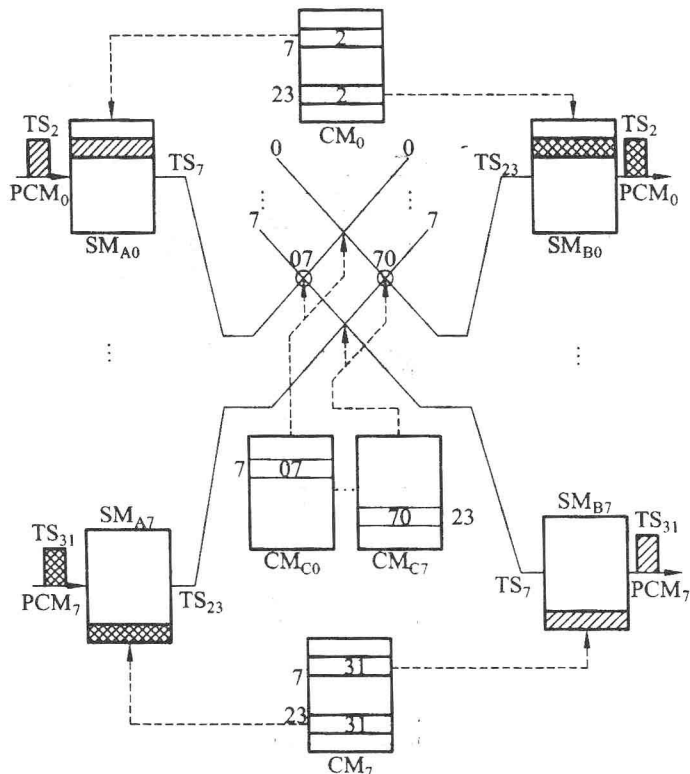
图 1.11 TST 网络结构图
