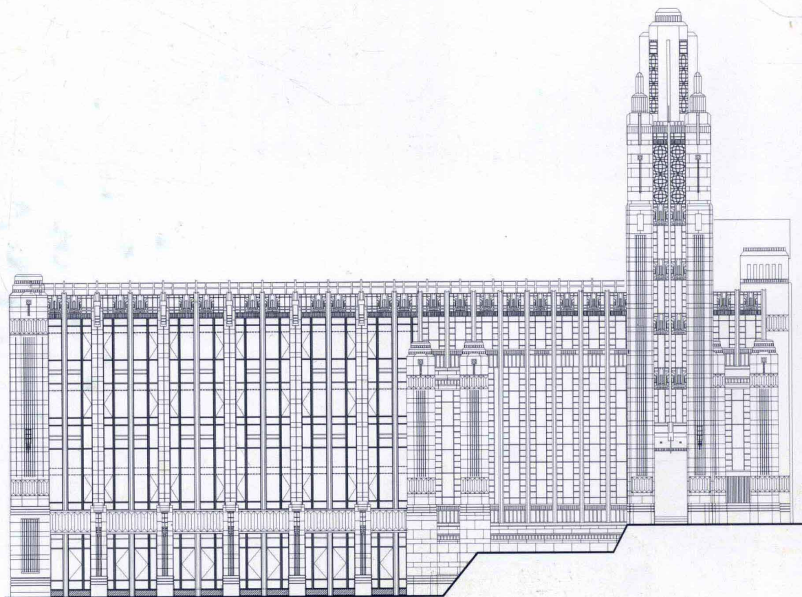
南立面图
