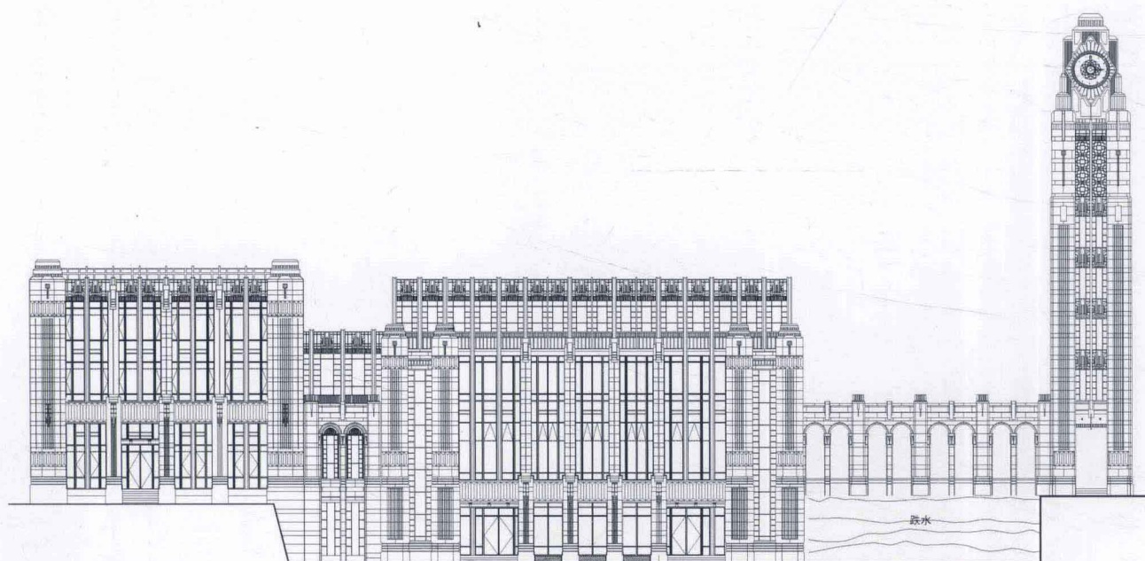
西立面图
