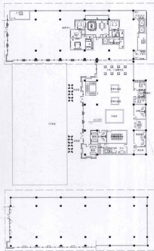
一层平面图
