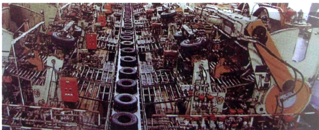
1979年，贵州轮胎厂。
