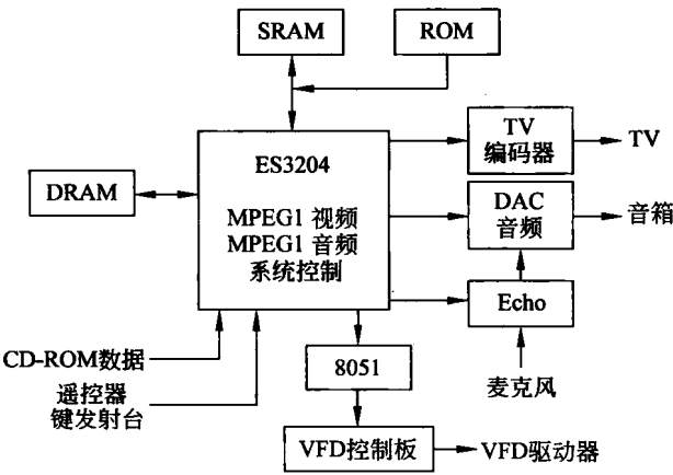
图 1.1 基于 ES-3204 芯片的 VCD 系统框图
