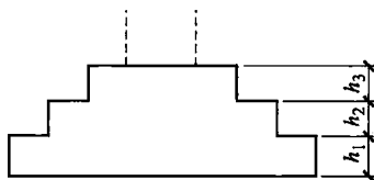
图 2-1 阶形截面普通独立基础 竖向尺寸注写方式
