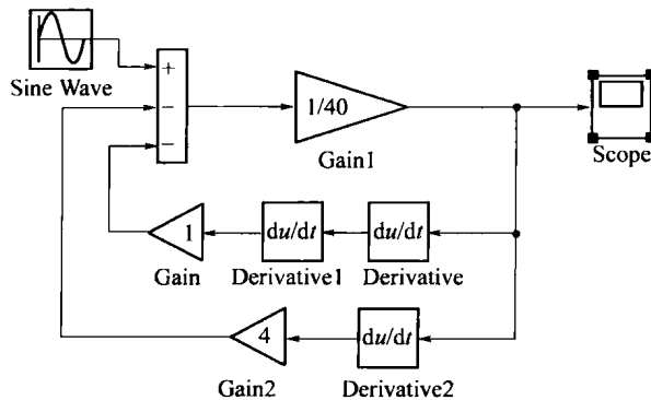
图 1-6 仿真框图 3
