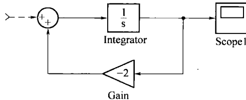
图 1-2 仿真框图
