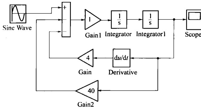
图 1-5 仿真框图 2
