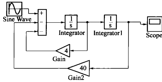
图 1-4 仿真框图 1
