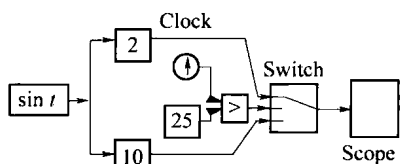
图 1-7 仿真示意图
