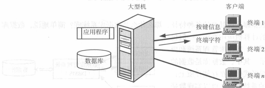
图1-4 大型机结构的数据访问模式
