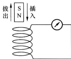
图 1-10 闭合电路在磁通量发生变化时会产生电流的实验
