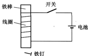
图 1-4 通电线圈产生磁场
