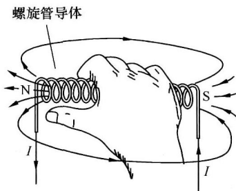
图 1-5 用右手螺旋定则判断通电螺旋管导体的磁场方向
