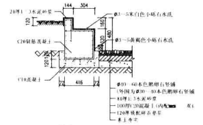
A-A剖面图
