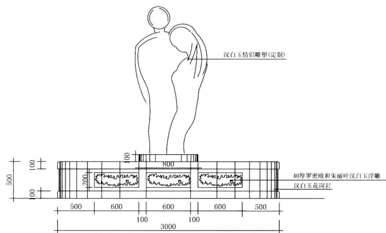
情侣广场花坛立面1:20
