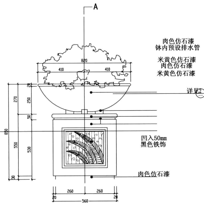
花钵大样图1:10
