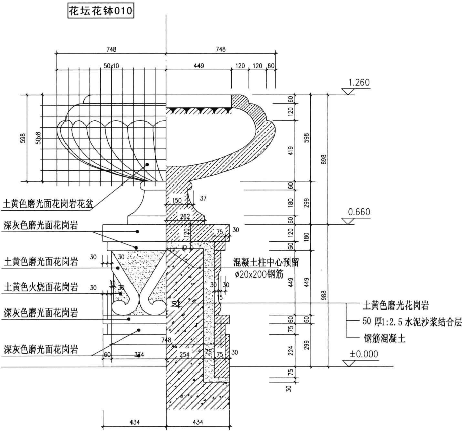
花钵详图1: 10
