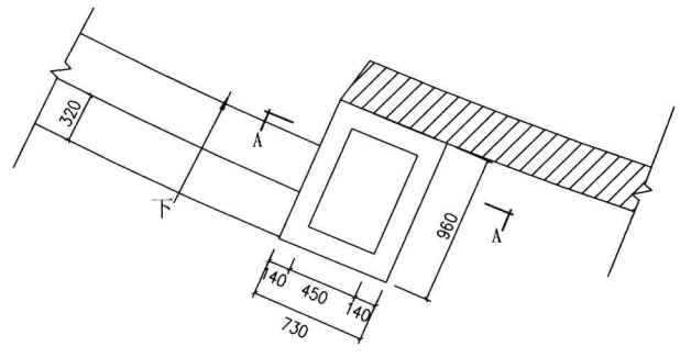
花坛平面图
