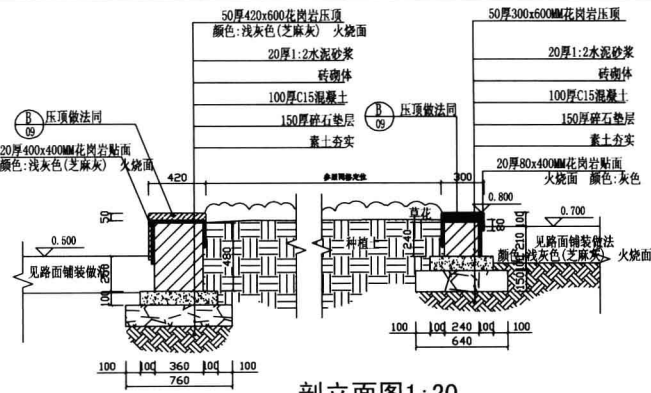
剖面图1:20
