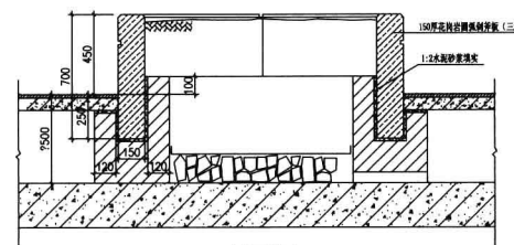
剖面图
