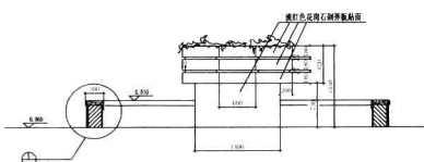
2-2剖面图
