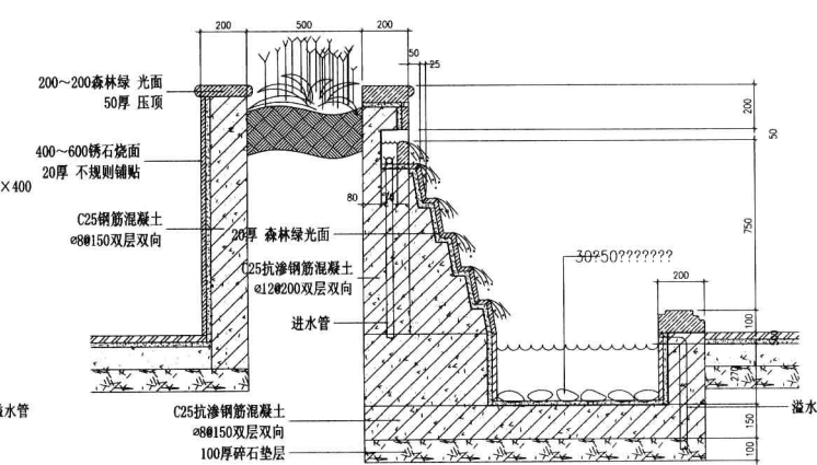
B-B 1:10
