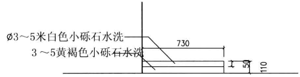
花坛立面图
