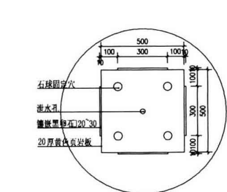
花钵平面1: 10
