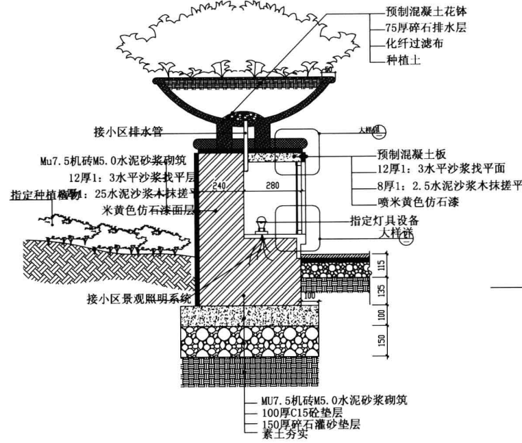
A-A断面图1:10
