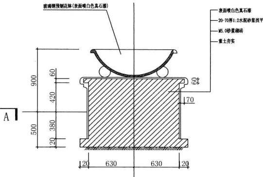
A-A剖面图1: 20
