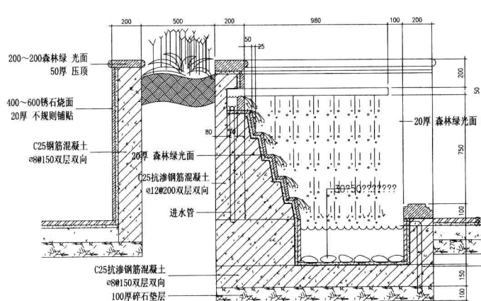
A-A 1:20
