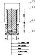
花坛剖面图
