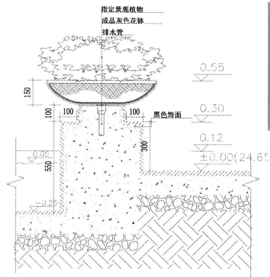
池边花钵剖面图1:15
