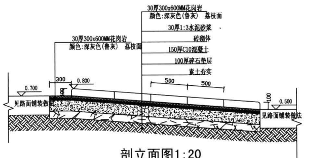
剖面图1:20
