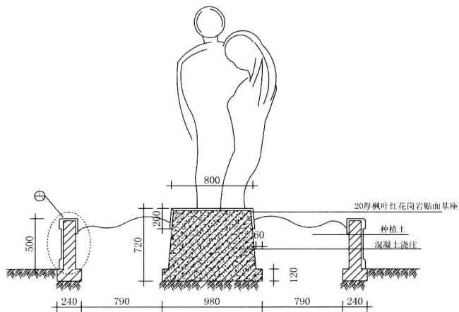
情侣广场花坛剖面1:20
