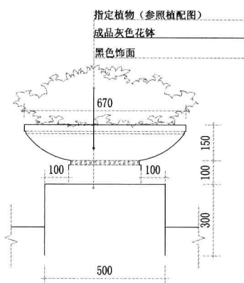
池边花钵立面图1:15
