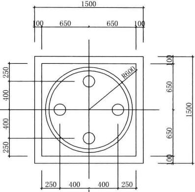
平面图1: 20
