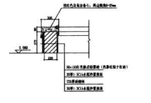
花坛壁剖面大样
