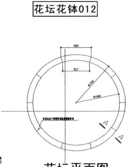
花坛平面图
