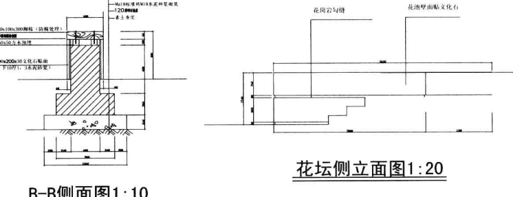
B-B侧面图1:10
