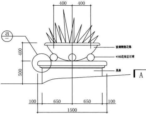
立面图1: 20
