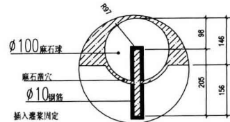
花钵节点1: 5
