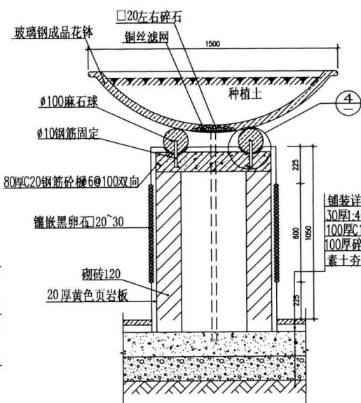
花钵剖面1: 10
