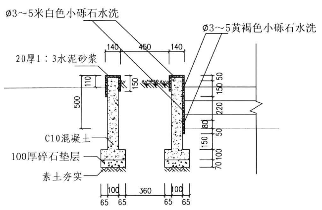
A-A剖面图
