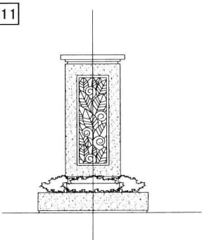
立面图
