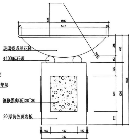
花钵立面1: 10
