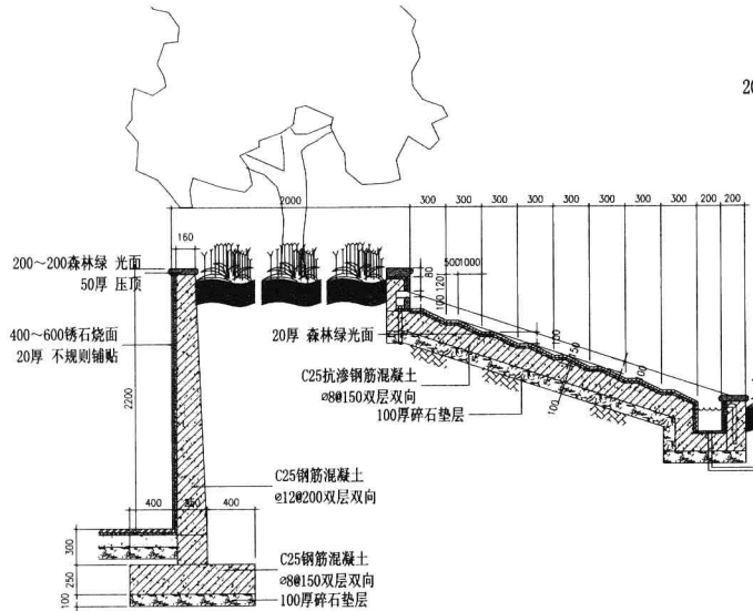
A-A 1:20
