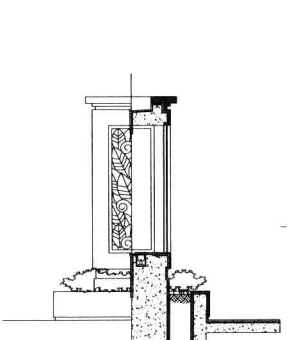
剖面图
