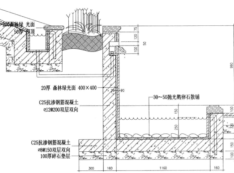
B-B 1:10
