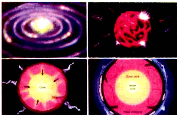
● 地球的形成过程示意图
