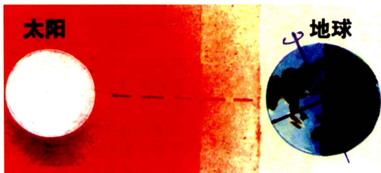
●地球昼夜形成示意图
