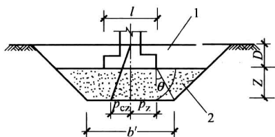
图 1-2 砂垫层内应力分布示意
