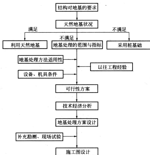
图 1-1 地基处理设计步骤
