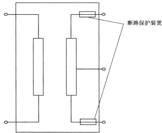
图 101 输出电路短路时的保护
