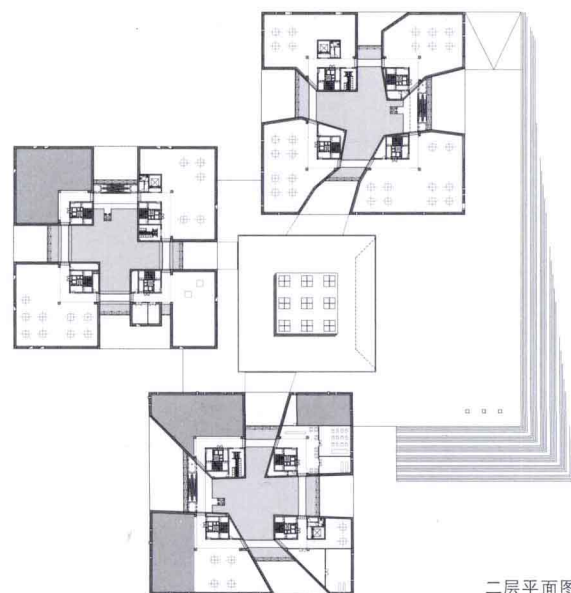
二层平面图
