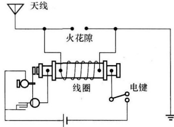
图 0-6 马可尼和他的无线电收发报机原理图
