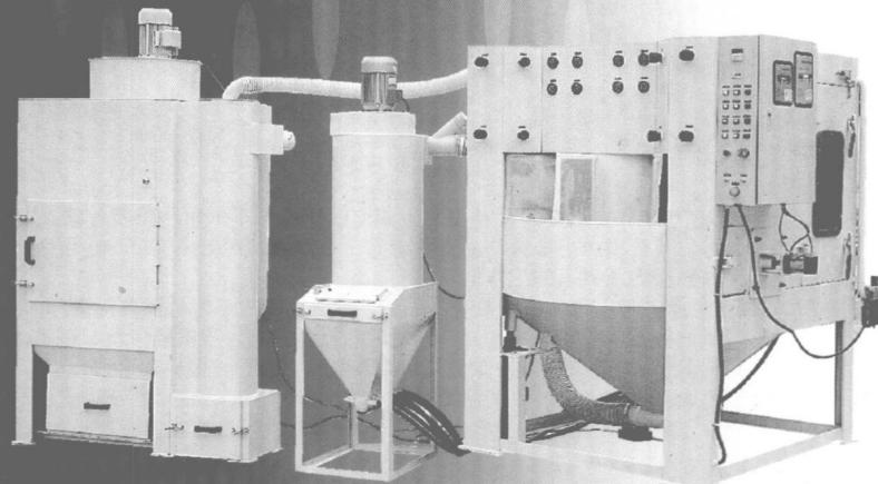
多工位自動回轉式噴砂機(適合于盤類，圓筒類零件批量生產)
