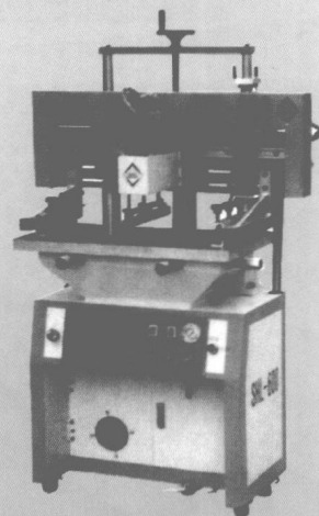
SHL800型电脑控制自动丝印机
