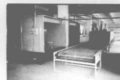
◆ 網帶噴塗線
