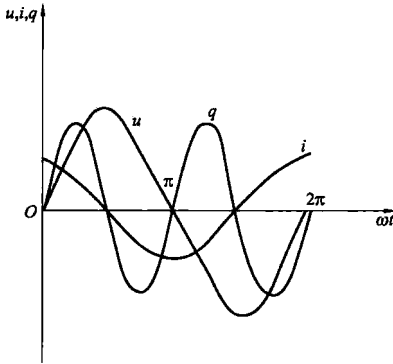
图 1-5 交流电容电路波形图
