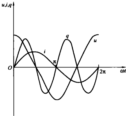
图 1-2 交流电感电路波形图
