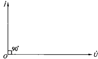
图 1-6 交流电容电路相量图
