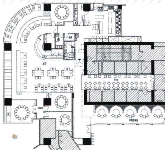
平面图
