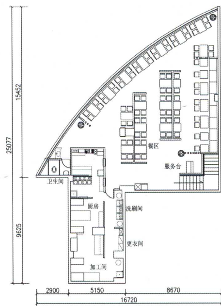
平面图
