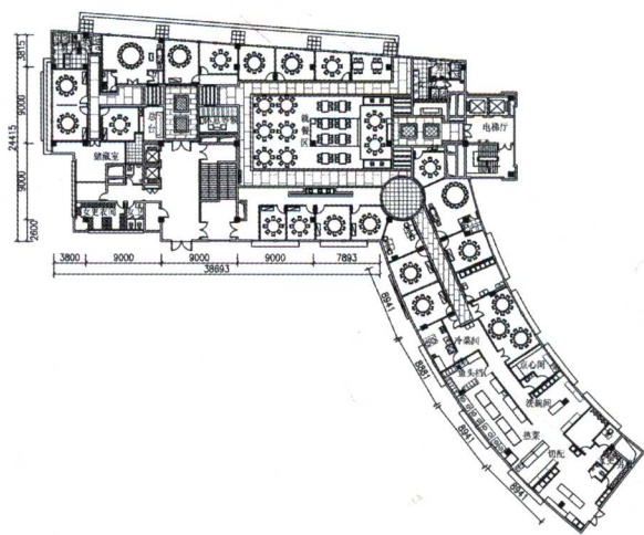
平面图
