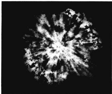
宇宙大爆炸
