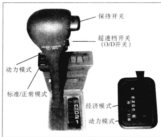
图 1-16 各控制开关
