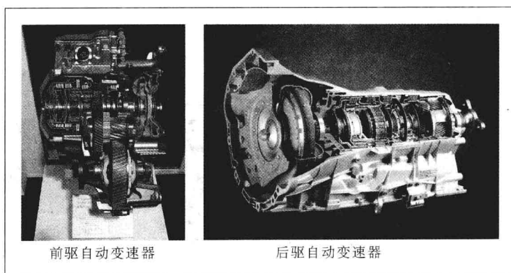
图 1-3 前、后驱自动变速器实物图
