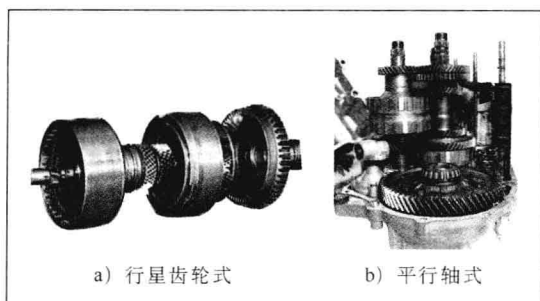
图 1-9 变速机构形式
