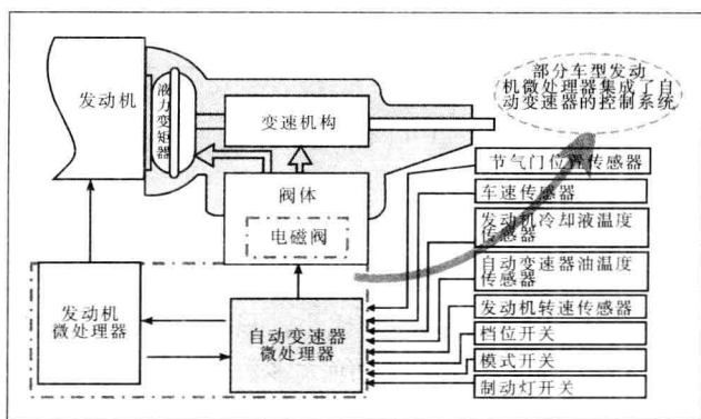
图 1-7 电控液力自动变速器系统简图
