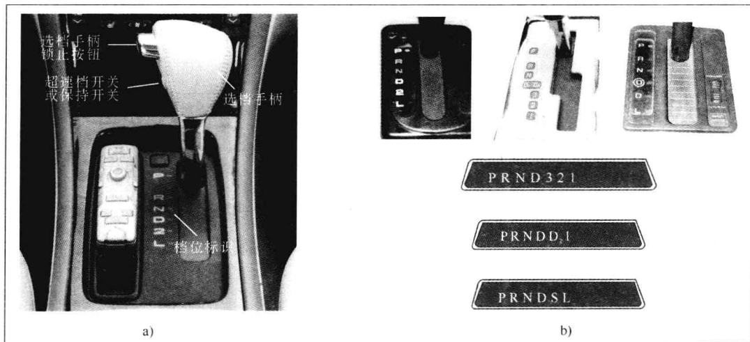
图 1-14 自动变速器选档手柄和档位指示器
