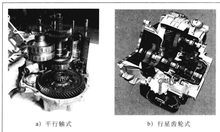
图 1-5 不同传动机构的自动变速器
