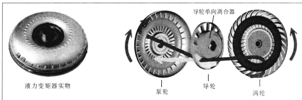
图 1-4 液力变矩器
