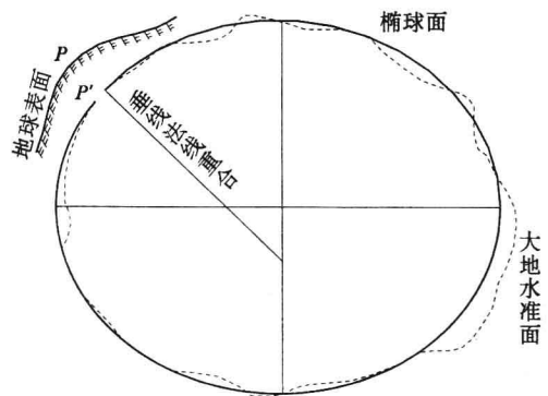
图 1-4 参考椭球体的定位
