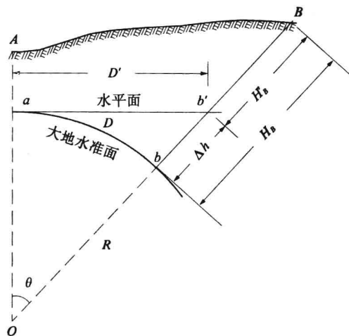
图 1-8 水平面与水准面的关系
