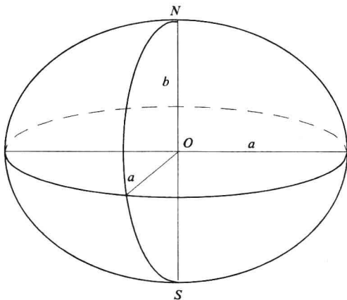
图 1-3 旋转椭球体
