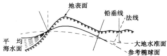
图 1-2 大地水准面
