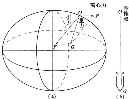
图 1-1 铅垂线方向
