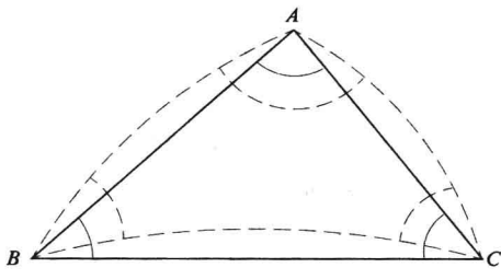
图 1-9 球面角超
