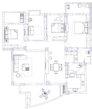
平面布置图
