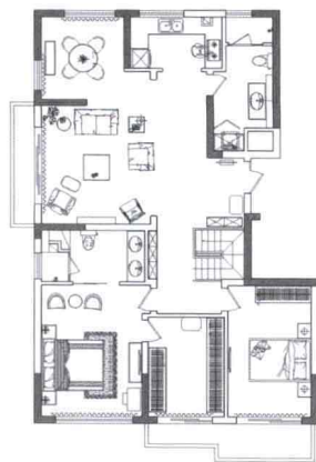
一层平面布置图
