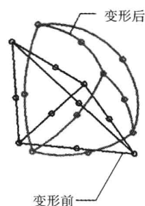
图 0-5 变形前后的二阶实体四面体单元
