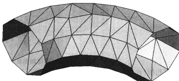
图 0-8 一阶三角形壳单元网格划分结果
