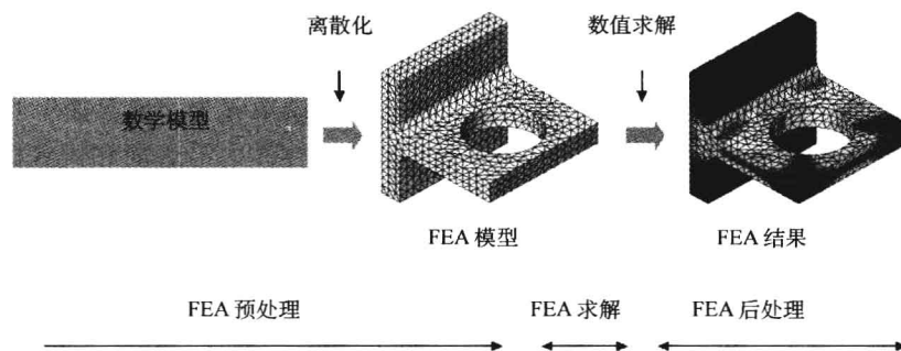
图 0-2 建立有限元模型的流程
