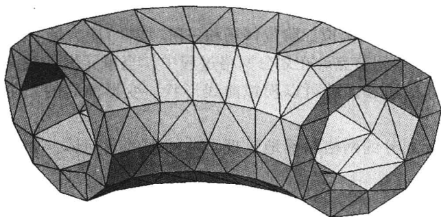
图 0-4 一阶实体四面体单元网格划分结果
