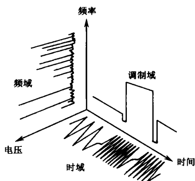
图 1.1 时域、频域和调制域
