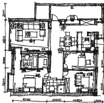
平面布置草图
