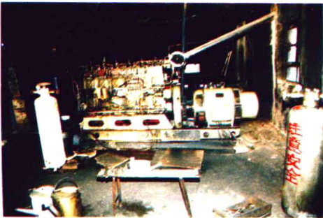
农九师170团庙尔沟柴油机 发电机组 (319千瓦)
