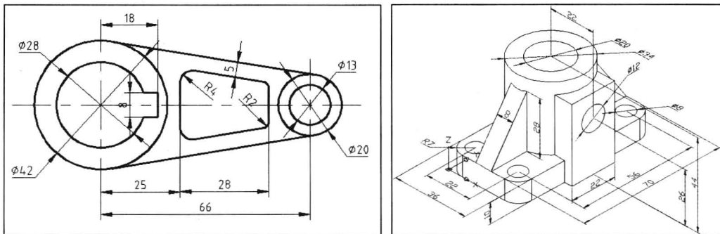
图 1-4 使用 AutoCAD 标注尺寸的二维图形和三维图形
