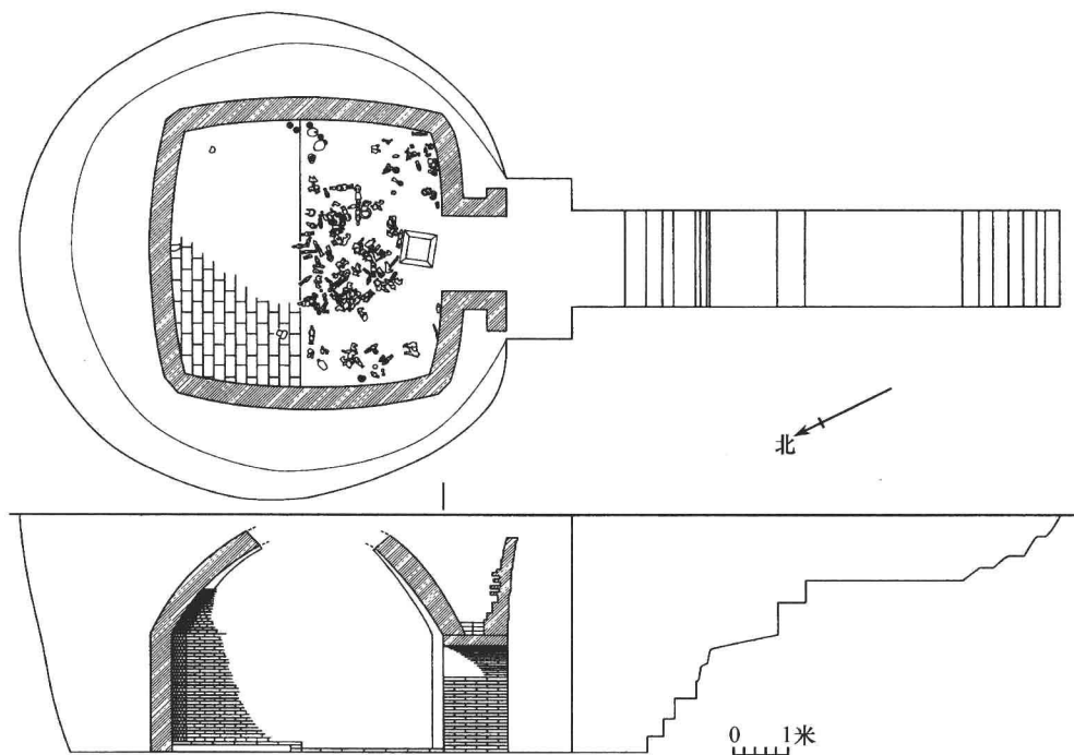
图一 墓葬平、剖面图
