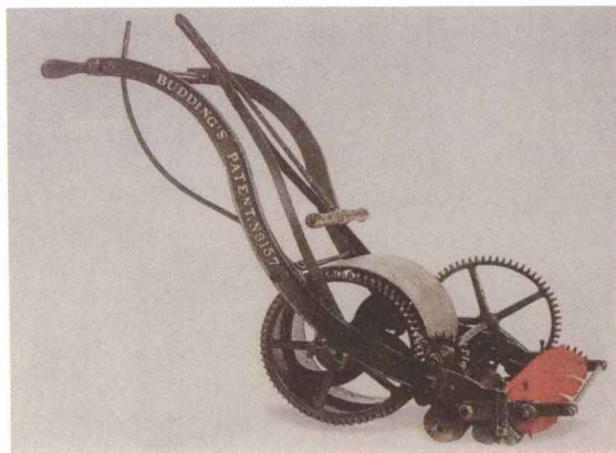
图55 埃德温·巴丁设计的世界第一台割草机，英国，1830年
