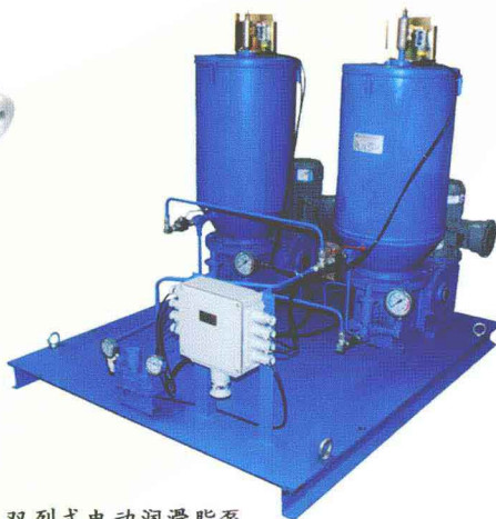
双列式电动润滑脂泵
