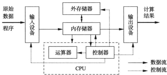
图 1-2 冯·诺依曼型计算机的基本结构
