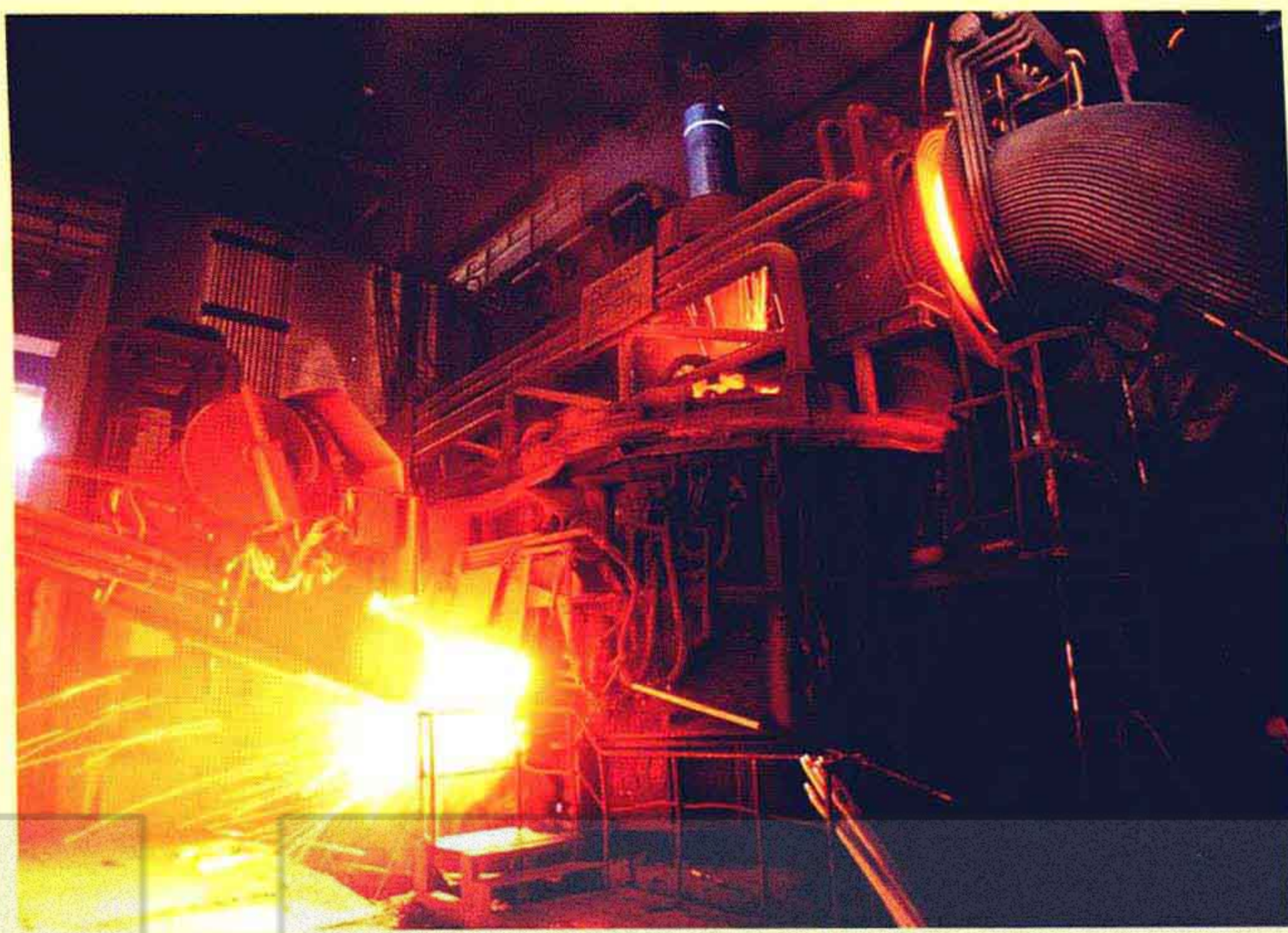
从德国德玛克公司引进的70吨超高功率直流电弧炉
