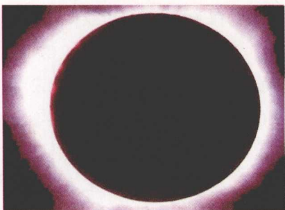
日冕
