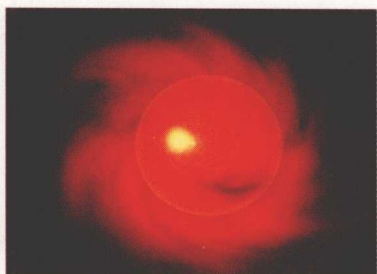
行星图
