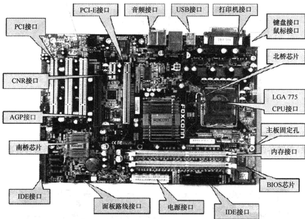
图 1-4 微机主板布局
