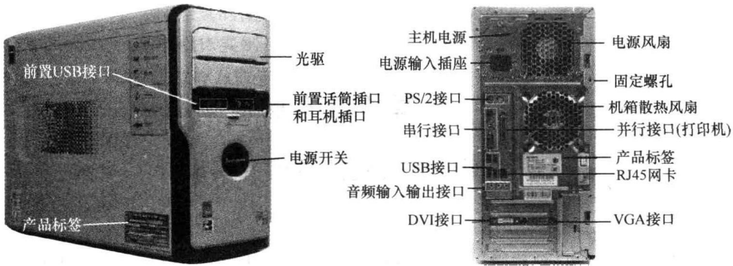
图 1-2 微机主机箱前面板和后面板外观图
