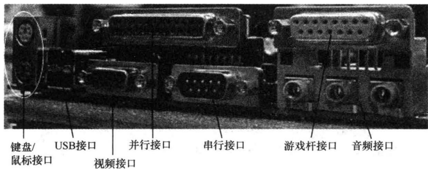
图 1-5 微机主机箱背板标准接口
