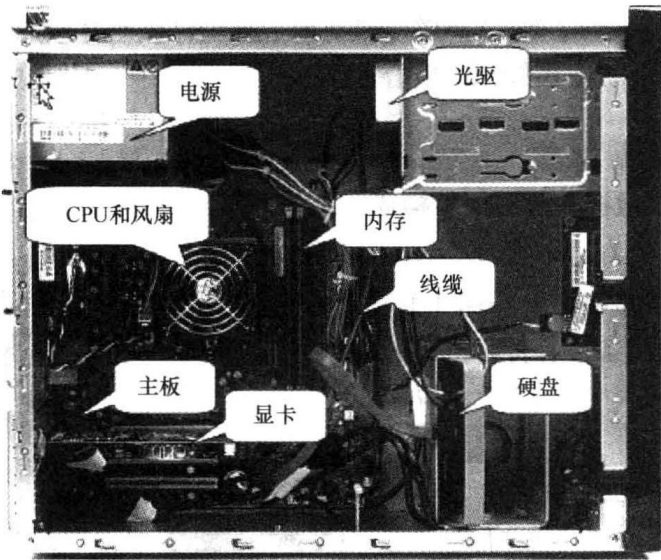
图 1-3 微机主机箱内部结构图
