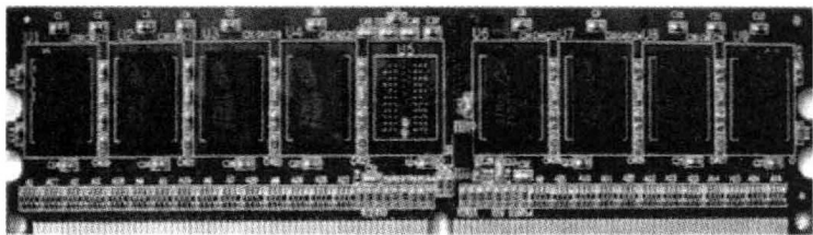
图 1-8 DDR-184 线内存条
