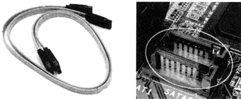
图 1-10 SATA 硬盘总线及接口
