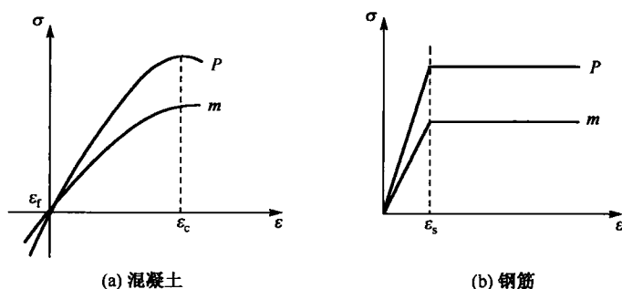
图 2.1 模型与原型应力-应变关系相似图
