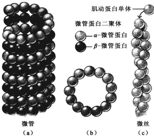
图 2-3 微管和微丝的结构
