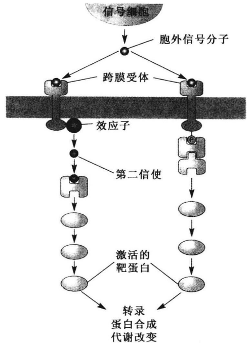
图 2-4 细胞信号转导途径
