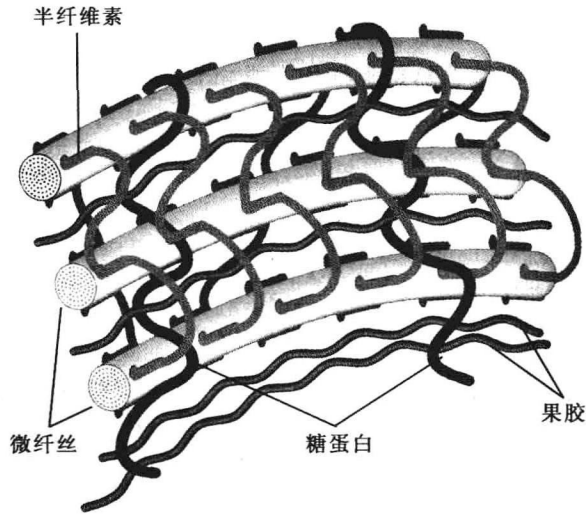
图 2-2 细胞壁分子组成模型 (Karp G, 2008)
