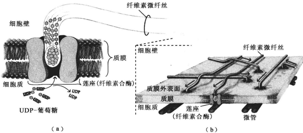
图 2-1 纤维素微纤维的合成(a)及其在细胞壁上的沉积(b)
