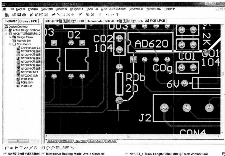
图 1-6 PCB 手动布线功能
