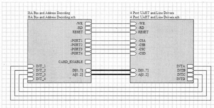
图 1-1 分层原理图的设计
