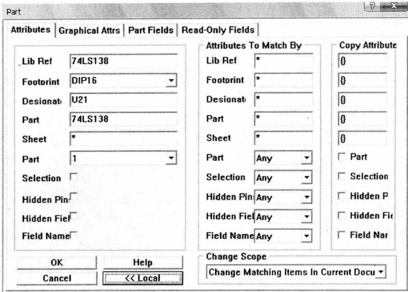
图 1-3 对象属性对话框和全局编辑功能
