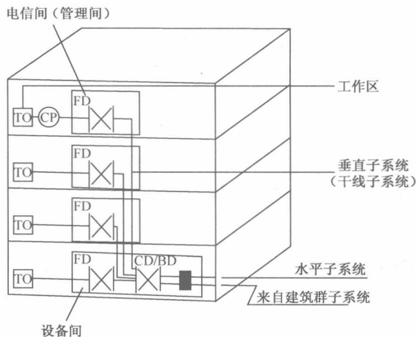
图 1-1 综合布线设备典型设置
