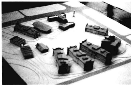
1/1000的工作模型用以探讨建筑物的布局及间距
