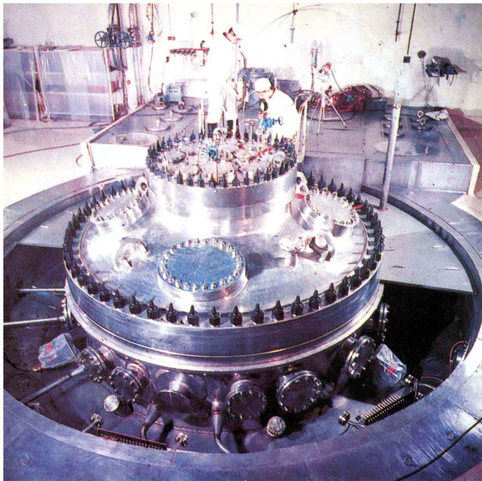
◀ 我国自行设计 建造的大型高通量 原子反应堆堆体
