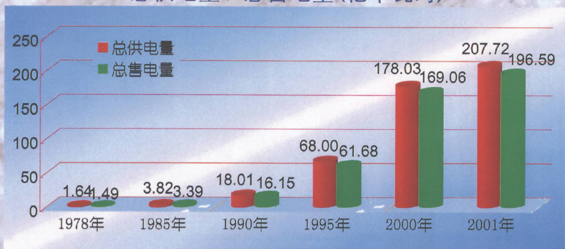
总供电量、总售电量(亿千瓦时)
