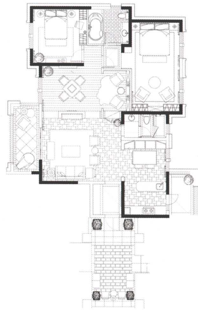
平面布置图
