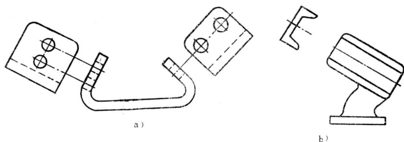
图1-12 JIS斜视图的画法(不加标注)
