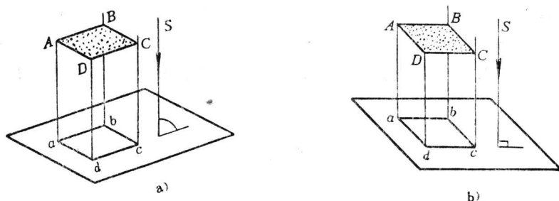
图1-2 平行投影法 a) 斜投影 b) 正投影
