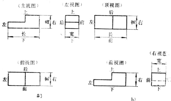
图1-8 两种投影中三视图对比
