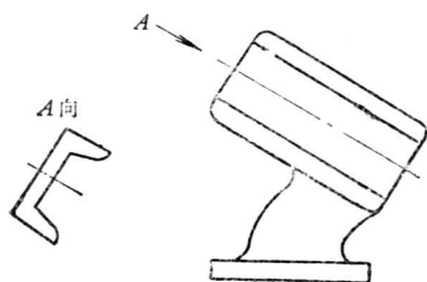
图1-13 JIS斜视图的画法(加标注)
