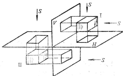
图1-4 第一角和第三角投影
