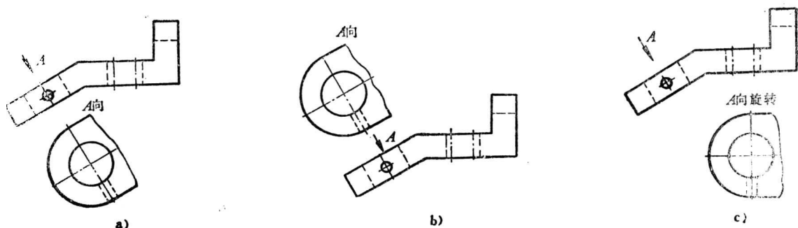
图1-11 GB斜视图规定画法
