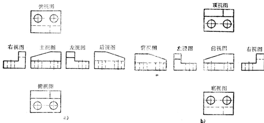
图1-10 两组基本视图
