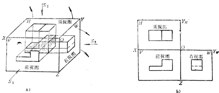
图1-7 第三角投影的展开及三视图
