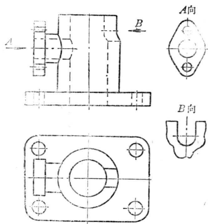
图1-15 GB局部视图的规定画法
