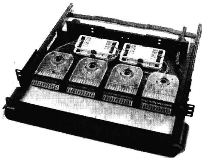
图 1-4 模块化光纤终端盒
