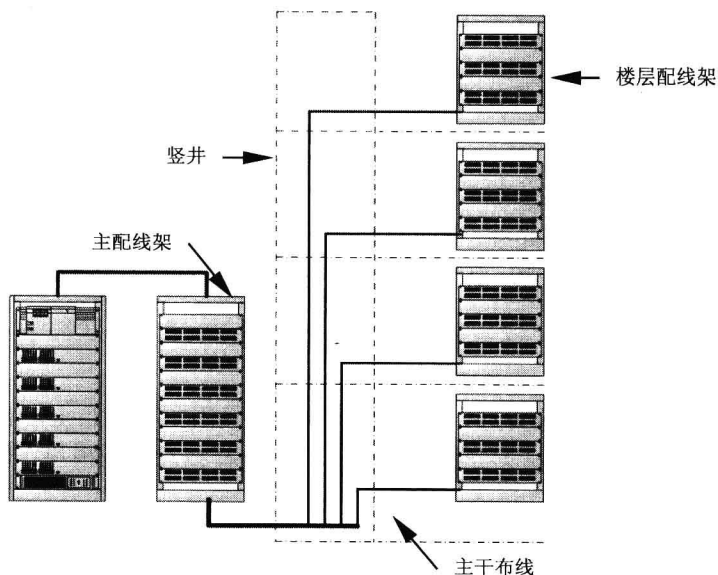
图 1-5 垂直主干子系统
