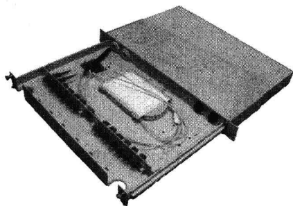
图 1-8 光缆配线架
