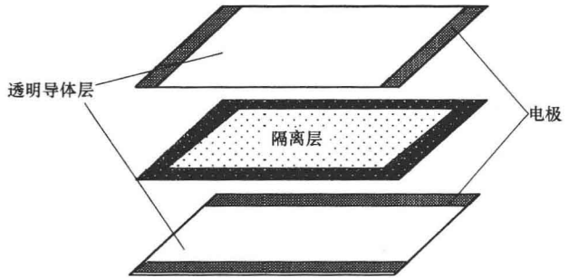
图 1-2 触摸屏结构
