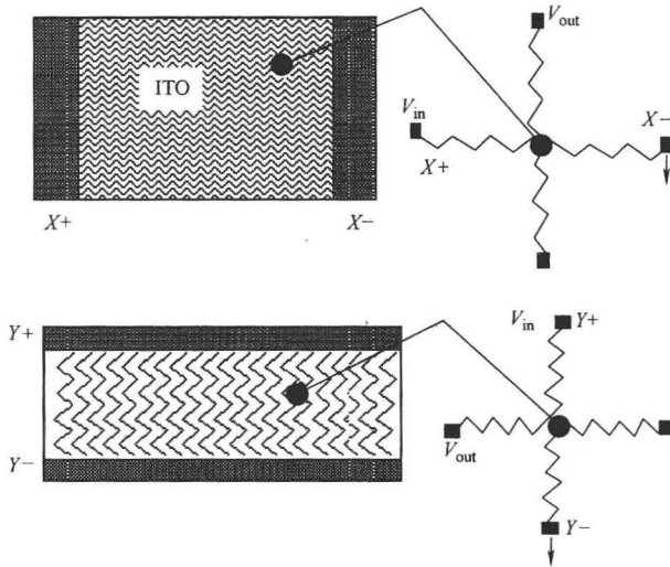
图 1-3 触摸屏下导体层的电阻网络
